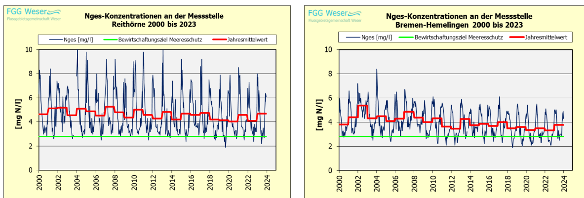
Abb. 5.2: Gesamtstickstoffkonzentrationen an den Referenzmessstellen für den Meeresschutz in der Flussgebietseinheit Weser (Stand: November 2024)
